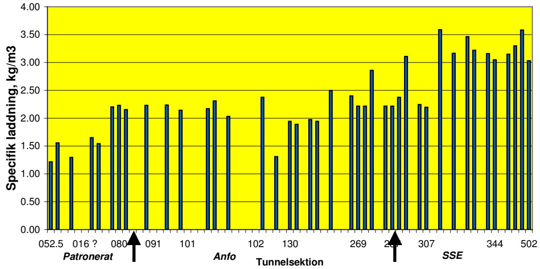
Diagram 10.1 Laddningskoncentration – Specifik laddning, kg/m 3
