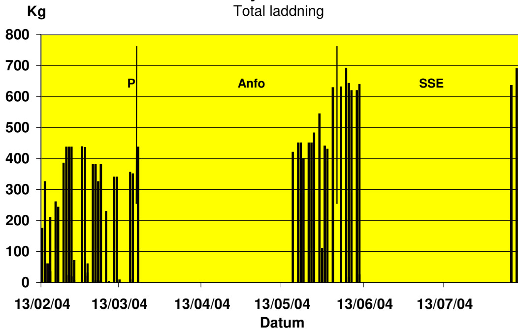
Diagram 10.2 Laddningsmängd – kg/salva
