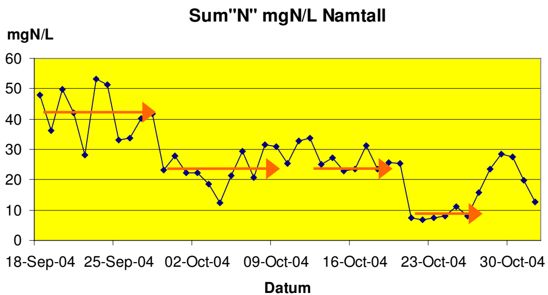
Diagram 9.1.6. Kvävemängd i processvatten – Namntall
