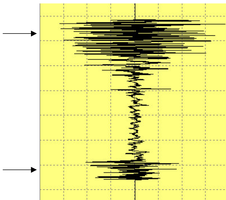
Figur 11.1. Kurva från luftstötståg – Höga värden i början och i slutet av kurvförloppet
